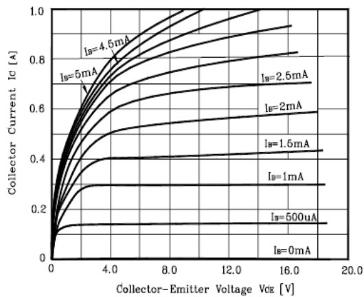
Fig. 5 I_C - V_{CE}
