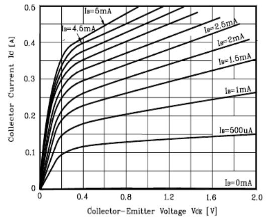
Fig. 4 I_C - V_{CE}
