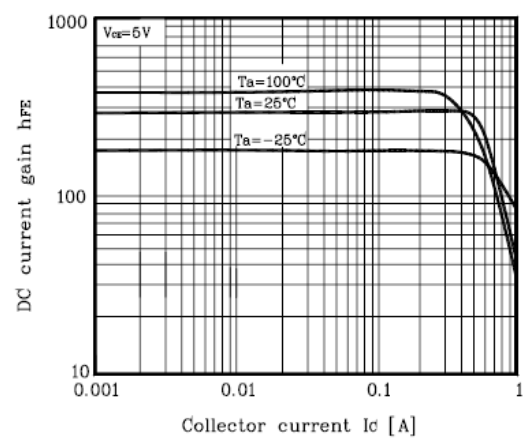
Fig. 6 h_{FE} - I_C
