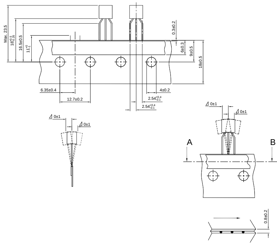
SECTION A-B
