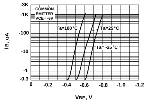
I_B - V_{BE}
