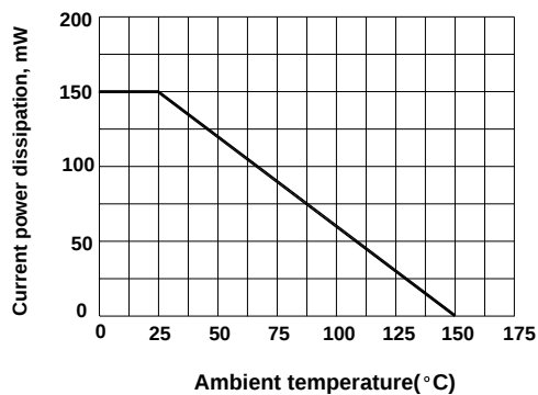
P_C - T_a
